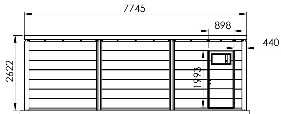
SECTION I-I SCALE 1 : 75
